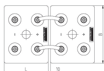
7 OPzS 700 bis 12 OPzS 1500
